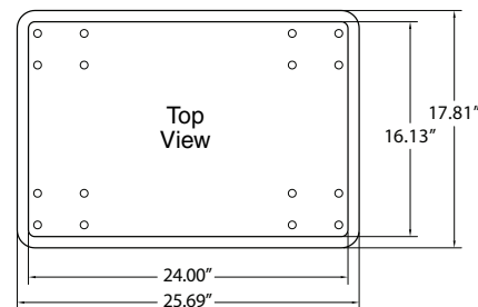
Dimensions - CSCD
