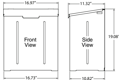
Dimensions - CSC
