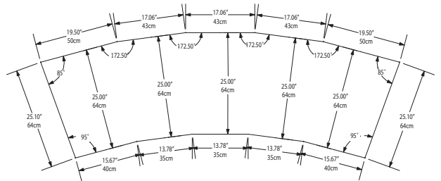
N8194-BR Cutout Dimensions
