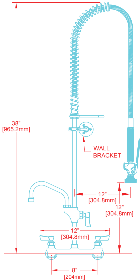
8" C/C BACKSPLASH FAUCET
