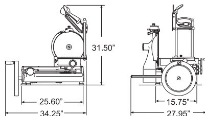
350VO / 370VO
