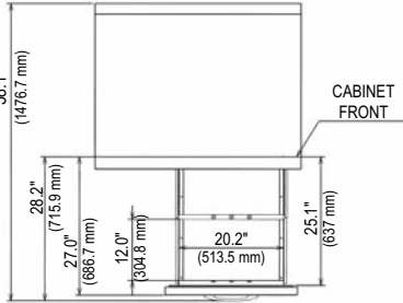
HWR40A-D (TOP VIEW)
