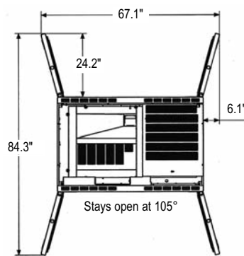
DOOR SWING
