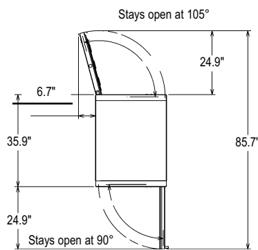
DOOR SWING
