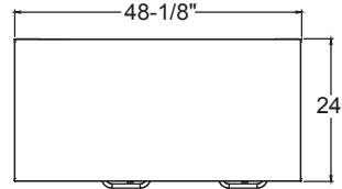
TOP NLBB48NG
