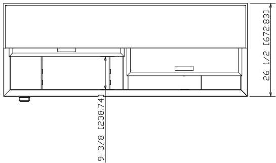
TOP NLBC69
