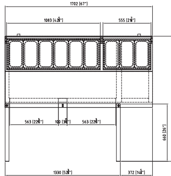
TOP VIEW FBPT67
