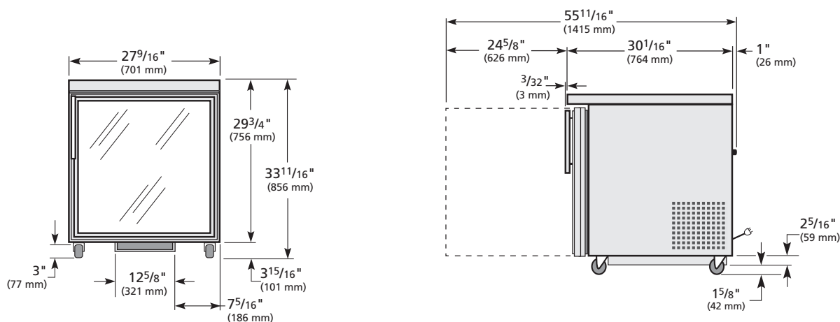
ELEVATION
