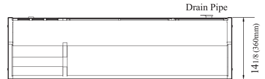
SAKURA-50R / SAKURA-50L TOP VIEW
